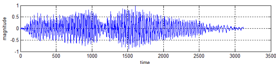
Gambar 3.Sinyal tutur “kiri” setelah proses HPF 200Hz
